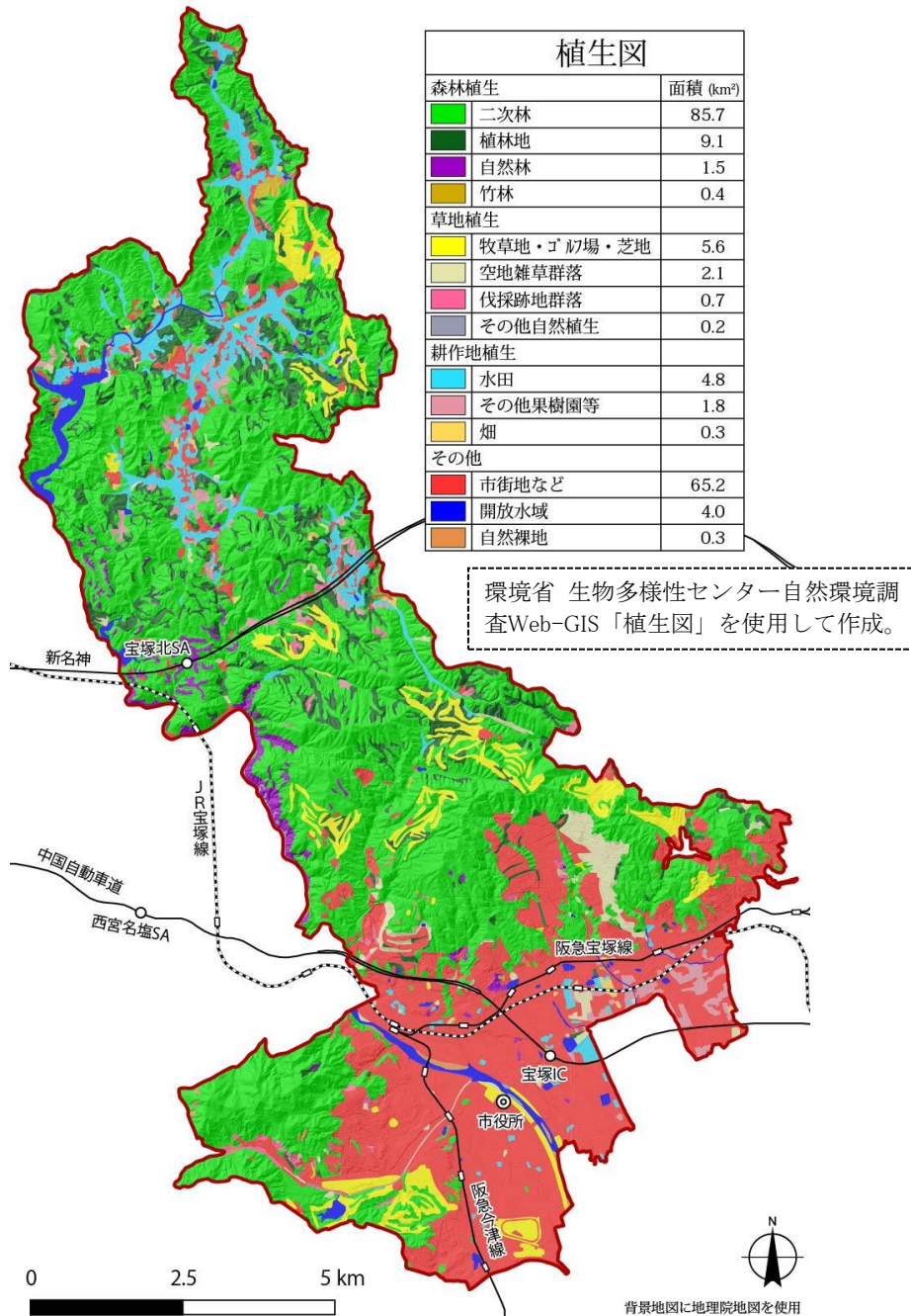
図2.1-14 植生の分布
