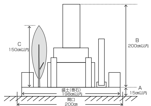
（例）普通墓所（長尾山霊園）墓石建立基準図（正面） （第１区～２３区 間口２ｍ・奥行き２ｍの場合）
