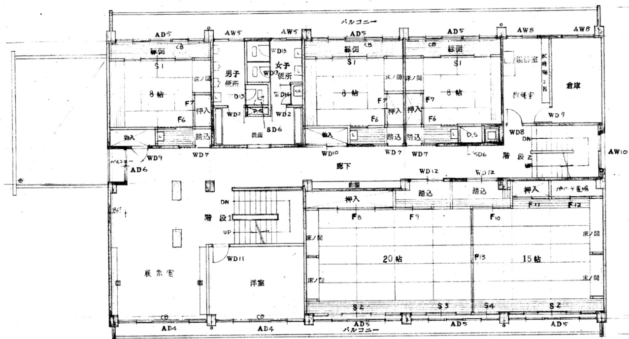
2 F 平面図
