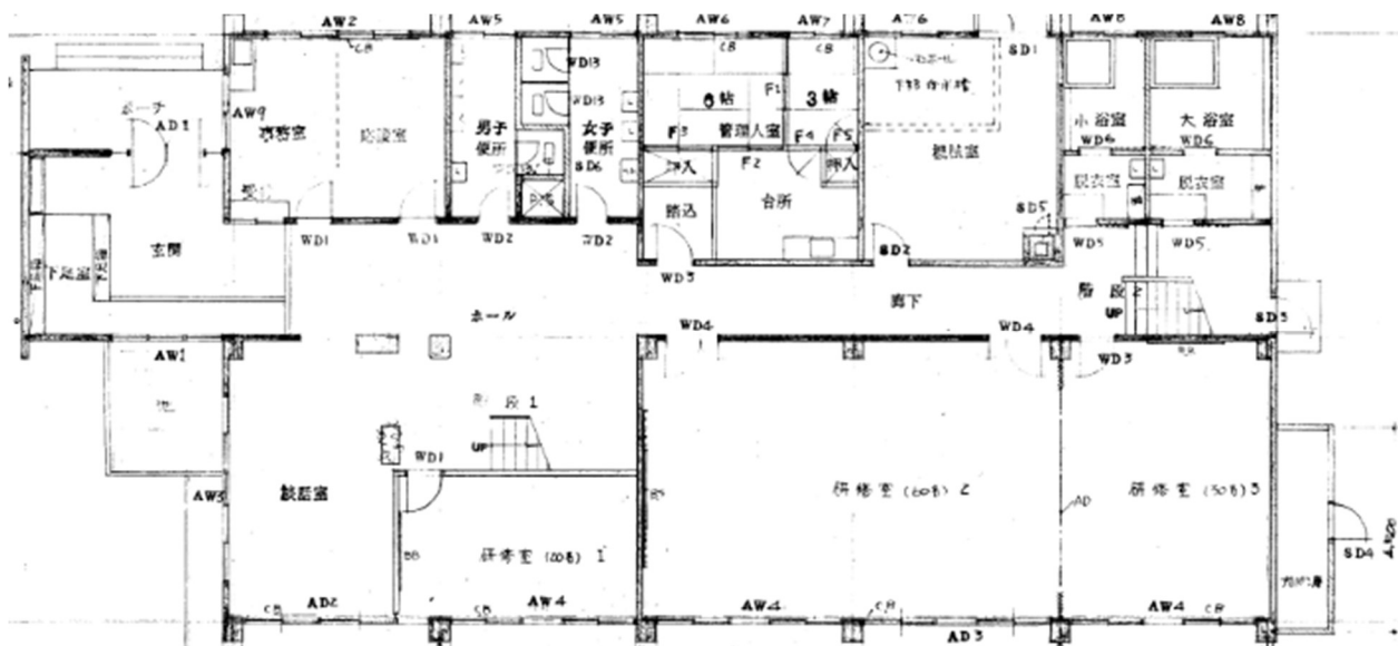
1 F 平面図
