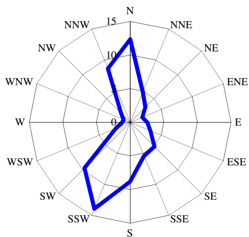
【図10】 西谷局風況図
