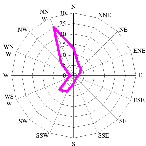
【図8】 高司中学校局風況図
