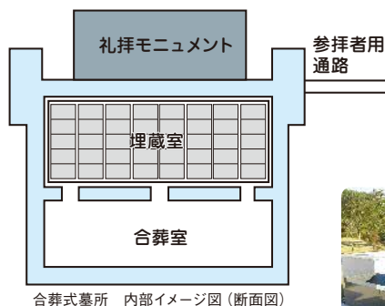
合葬式墓所 内部イメージ図(断面図)
