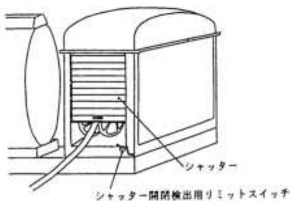
図 4-2-3 給油設備の扉による方法
