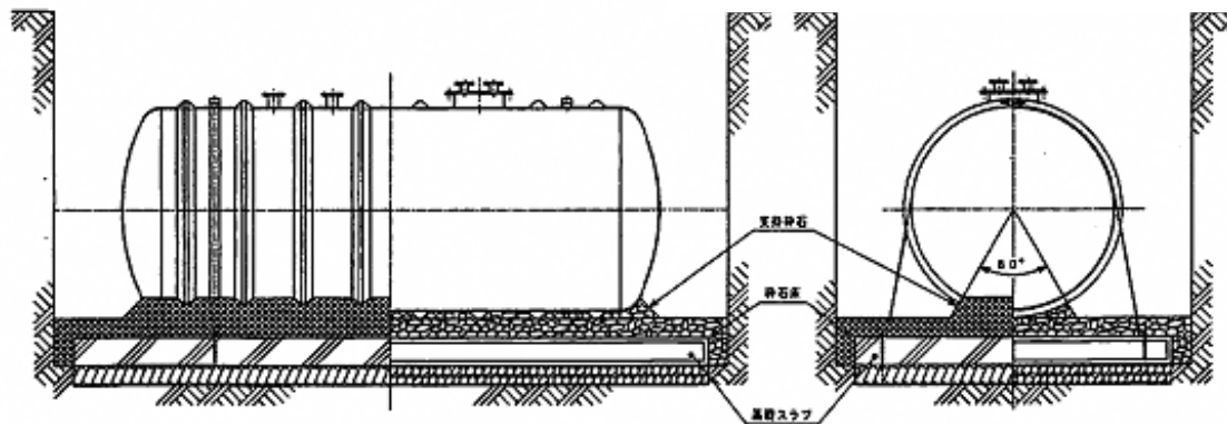
図7-2 支持碎石施工図
