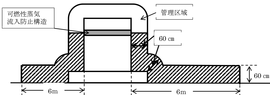
b 地上式固定給油設備（可燃性蒸気流入防止構造付き）
