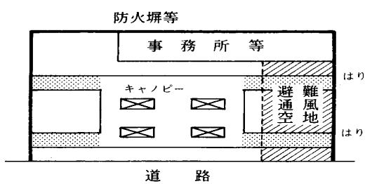
空地の上方にはりがある場合
