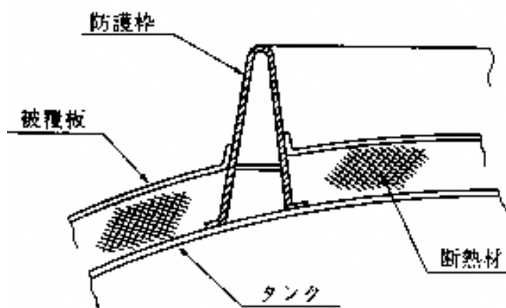
図 2-8-6 タンク銅板に直接取り付ける防護枠
