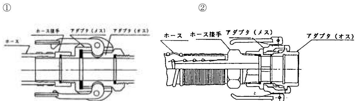
図 2-14-1 突合せ固定式結合金具の構造例
