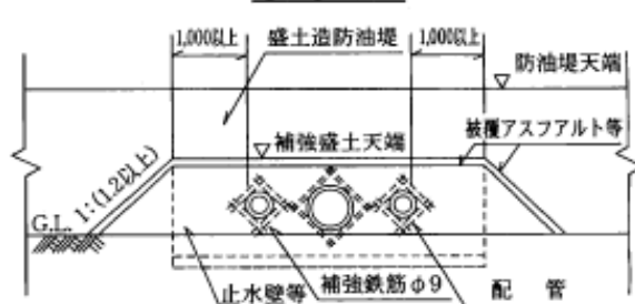
①—①断面図
