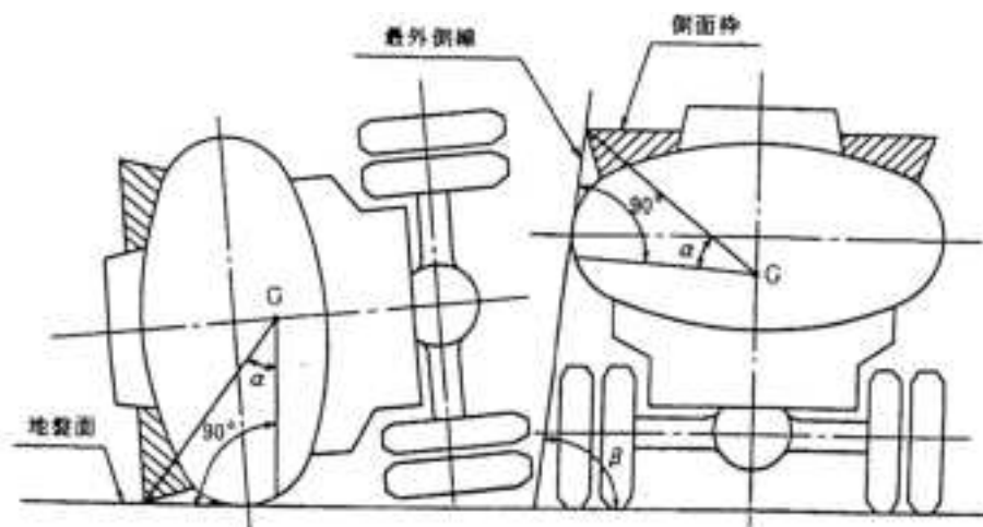
図2-7-6 接地角度及び取付角度
