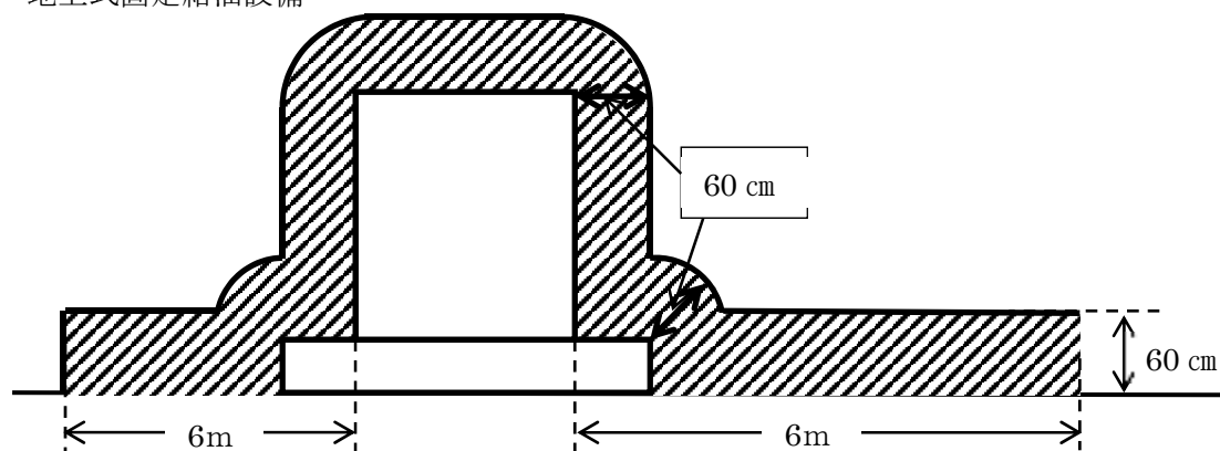
a 地上式固定給油設備
