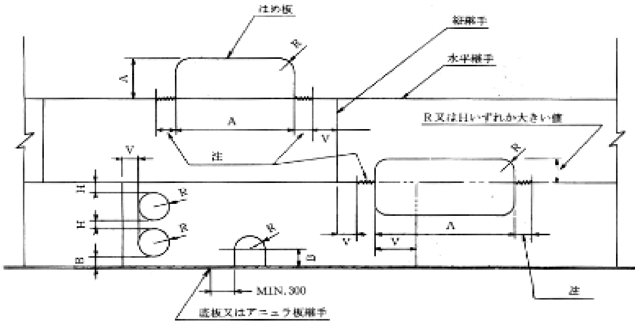
図 5 側板のはめ板取付け
