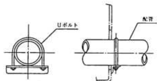
図 2-11-1 吐出口付近の配管の固定方法
