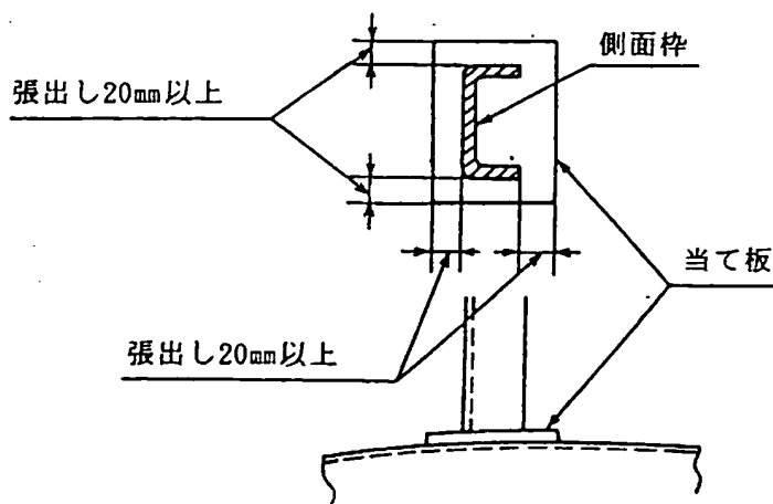
図 2-7-3 枠形の側面枠に設ける当て板の取付方法
