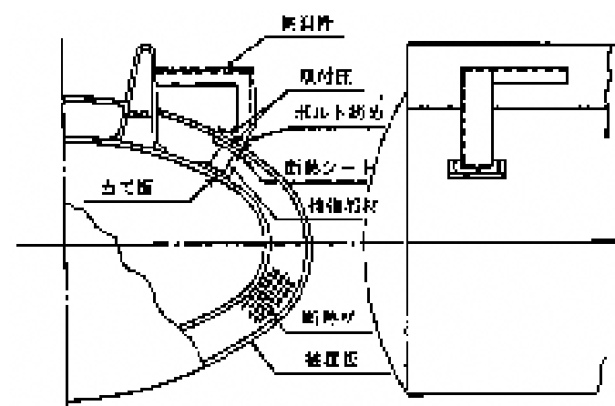
図 2-7-10 外板の下部に補強部材を設け、側面枠と補強部材をボルト締めにより接合する場合
