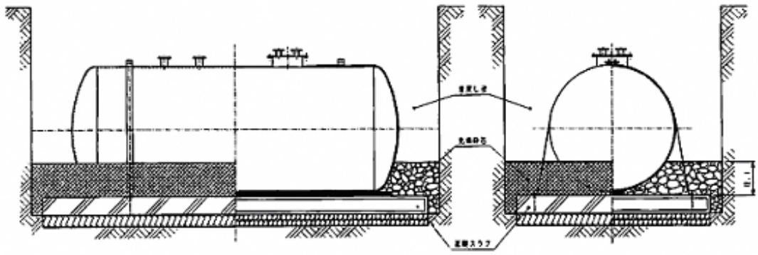
図8-2 充填碎石施工図
