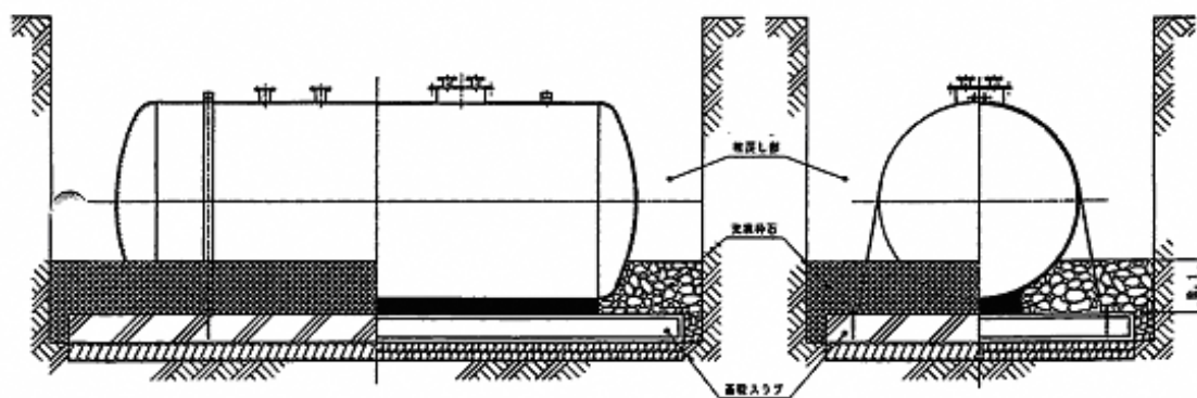
図9-1 充填碎石施工図
