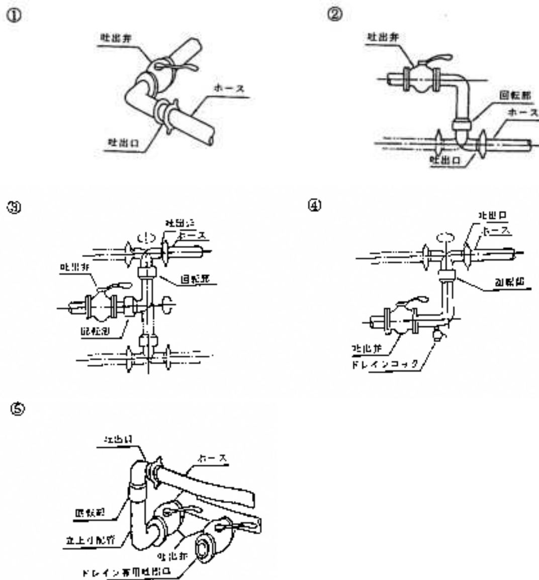
図 2-14-2 配管先端部の構造
