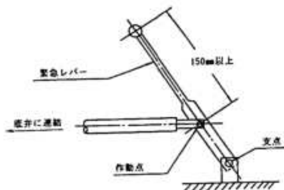
図2-10-1 緊急レバーの構造
