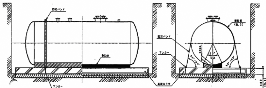
図9-1 碎石床施工図
