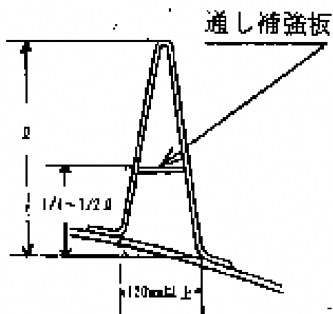
図 2-8-3 防護枠の通し板補強構造
