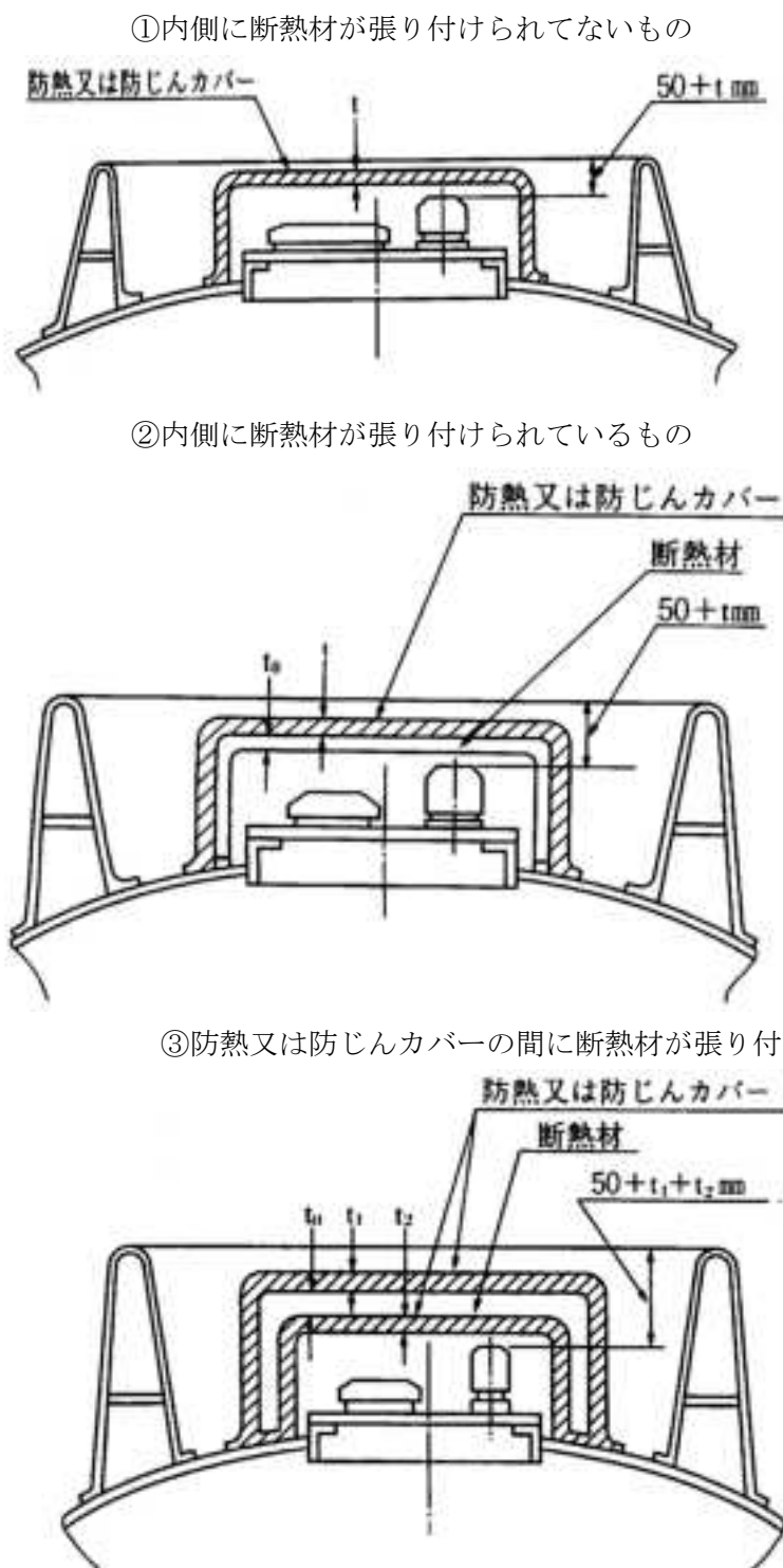
図 2-8-4 防熱又は防じんカバーを設ける移動貯蔵タンクの防護枠
