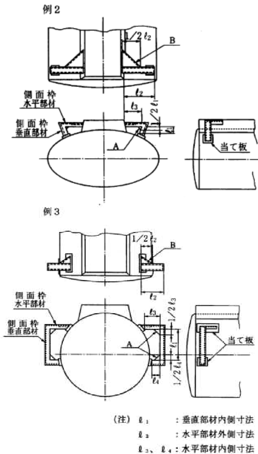
図 2-7-1 枠形の側面枠の構造
