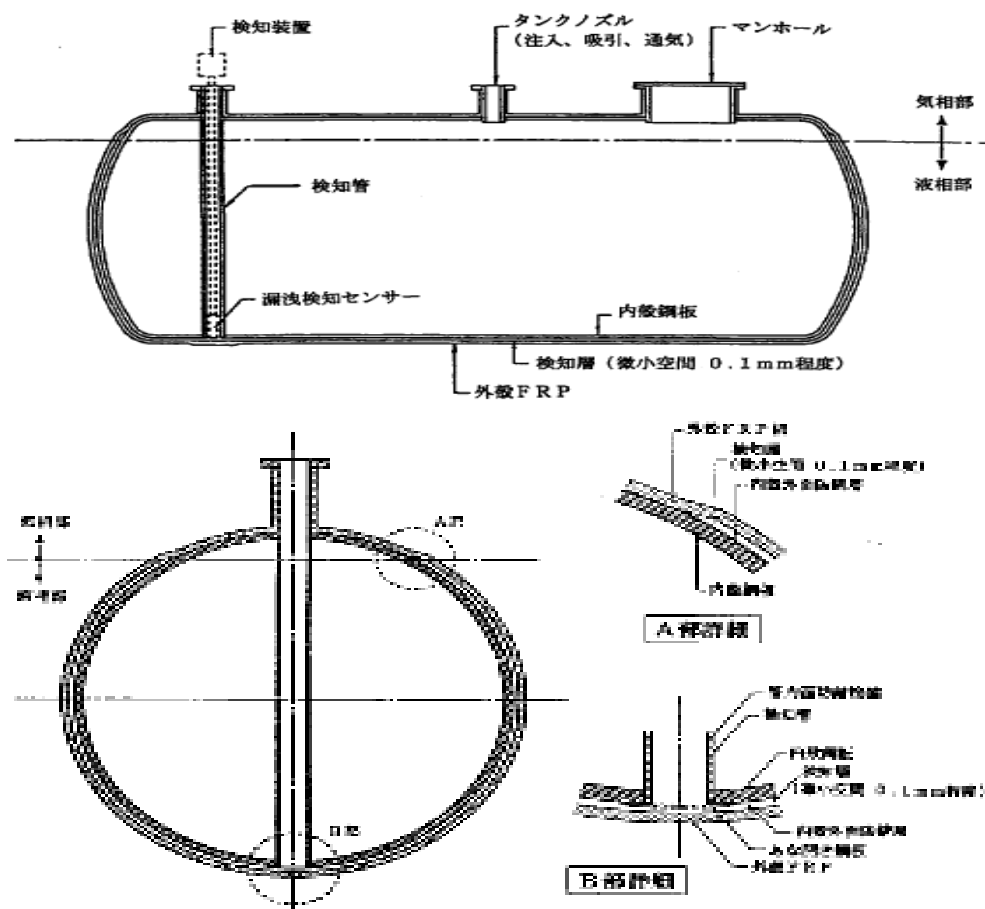
図3 SF 二重殻タンクの構造例
