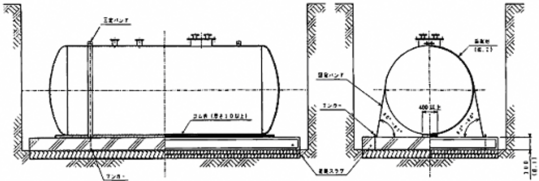
図8-1 碎石床施工図
