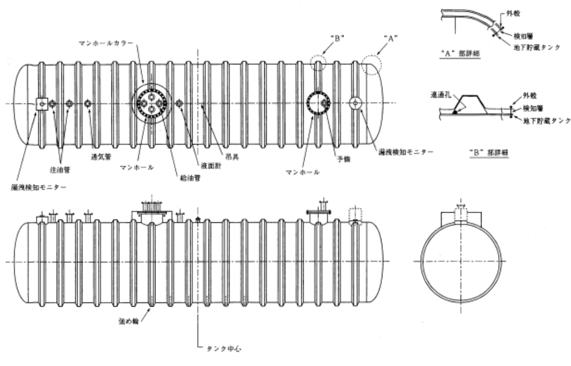
図6 FF 二重殻タンクの構造例
