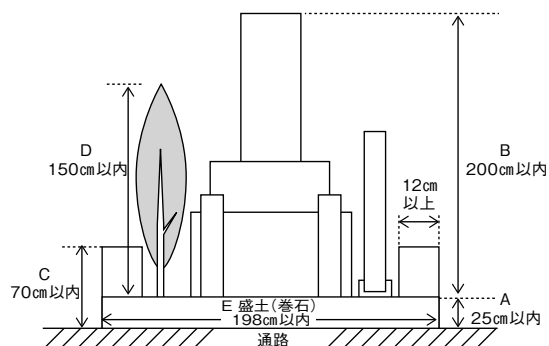
一般区域(すみれ墓苑)墓石建立基準図 (4平方メートルの場合)
